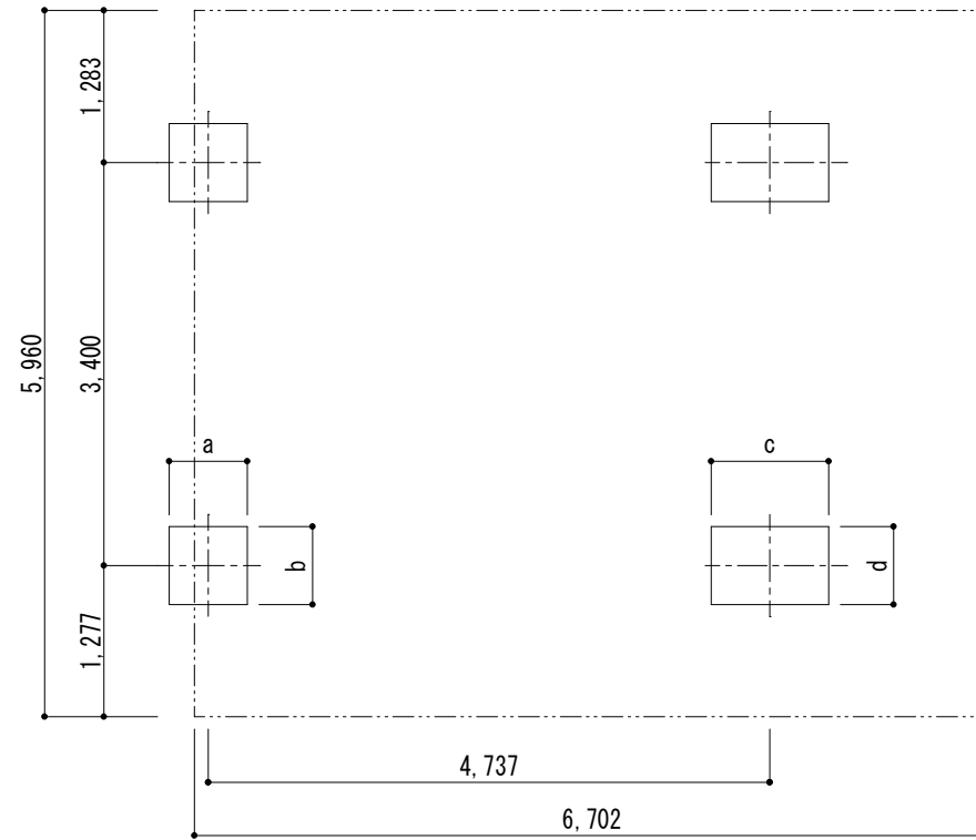
■ 基礎配置図
